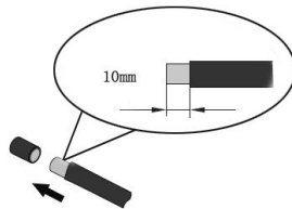
图 3.11 加工线缆
