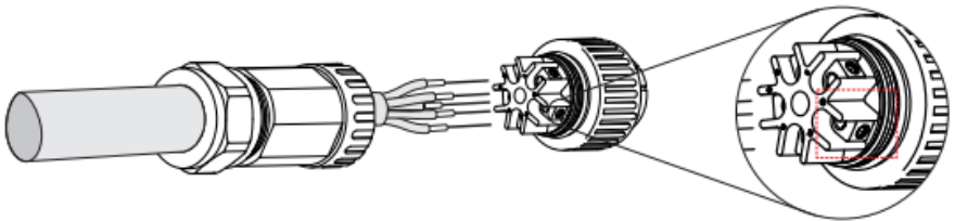
图 3.12 连接电缆线
